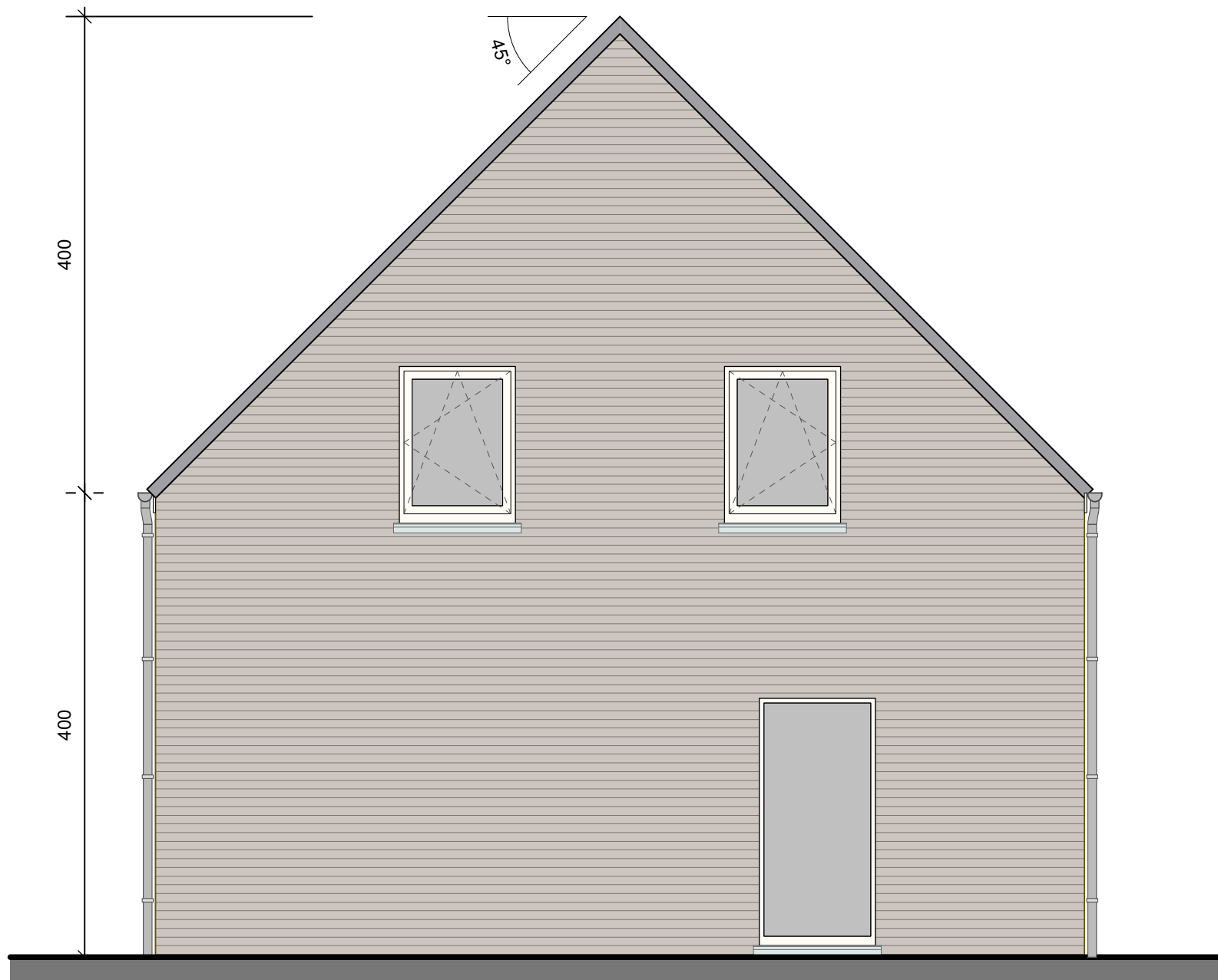
Zijgevel rechts
